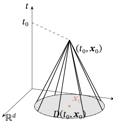
图 2.9: 顶点为 (t_0, \mathbf{x}_0) 的特征锥示意图
