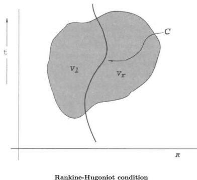
图 1.5: Rankine-Hugoniot条件示意图
